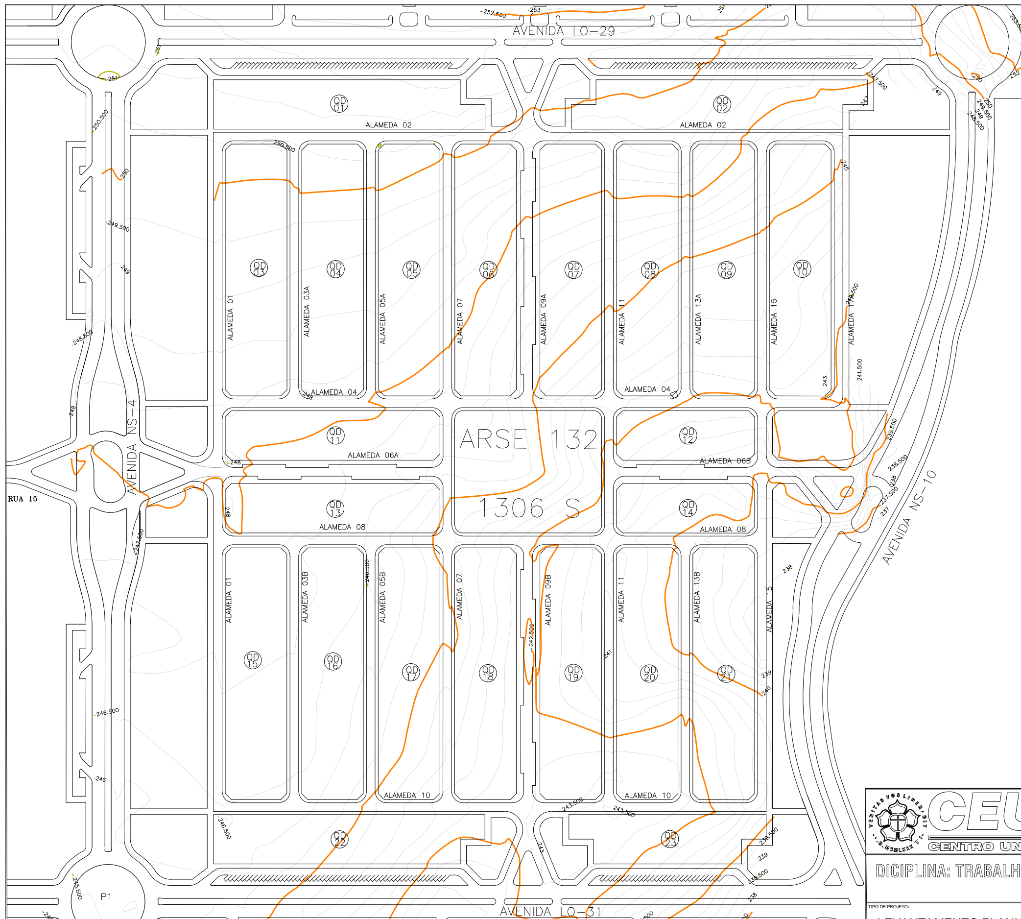
Planta do Levantamento Topografico Escala: 1 / 3.000
