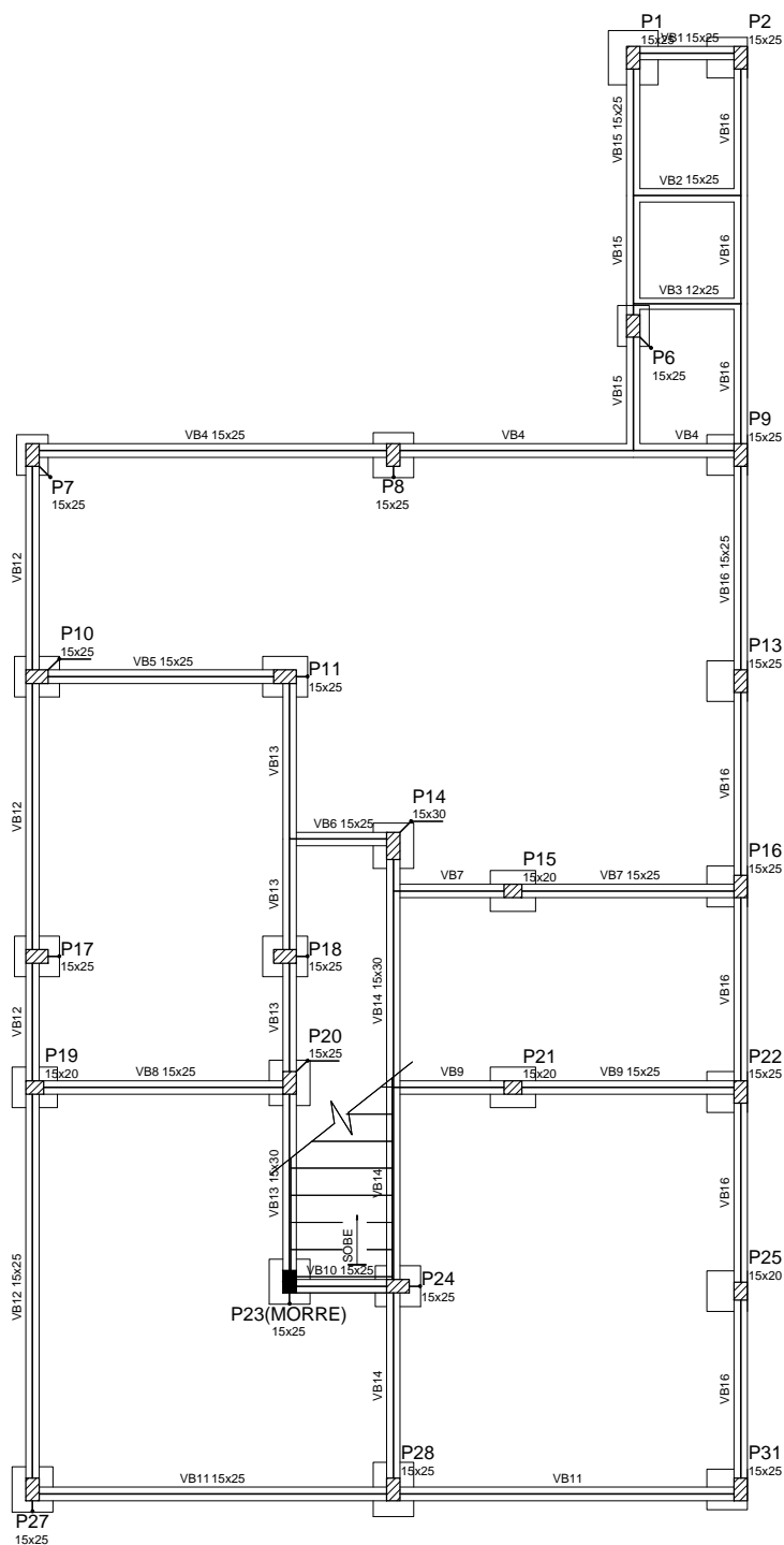
Forma do pavimento BALDRAME
