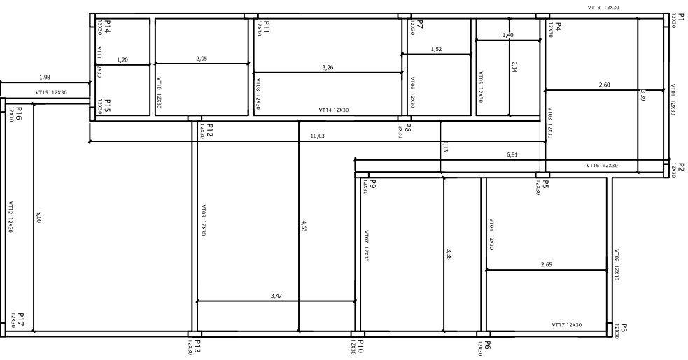
PLANTA DE FORMA SUPERIOR ESCALA 1:75
